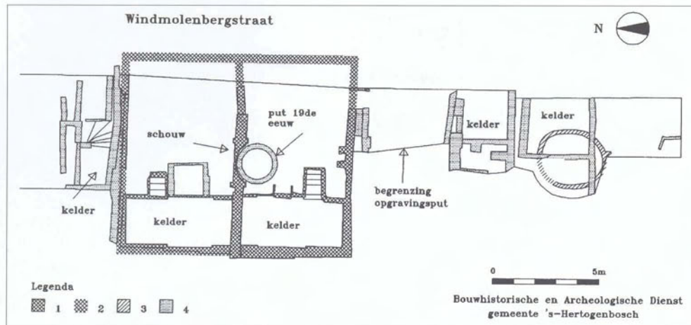
Afb. 2. Het opgegraven muurwerk langs de Windmolenbergstraat. 1) 2/1-kap-huis, midden 15de eeuw; 2) reconstructie 2/1-kap-huis; 3) beerput, 16de eeuw; 4) overig muurwerk, 14de-19de eeuw. (Tekening: F. Schipper, BAD)
