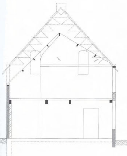
Afb. 2. Doorsnede over Putgang nr. 8 met aanzicht van de voormalige eindgevel, reconstructie van de voormalige geveltop. Op de begane grond de restanten van een voormalige zijdeur, rechts op de (zolder-) verdieping een dichtgemetseld venster uit de 17de-eeuwse fase. (Tekening: J. v.d. Eerden jr., BAD)
